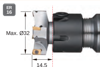
Ergo - Wendeschneidplattenfräser
