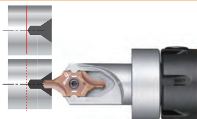
Ergo - Wendeschneidplattenfräser
