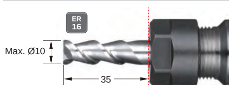
Vollhartmetall - Schaftfräser
