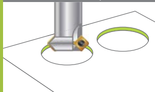
Конический зенкер
